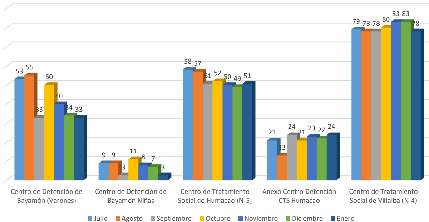
Comparación Promedio Mensual por Centro
